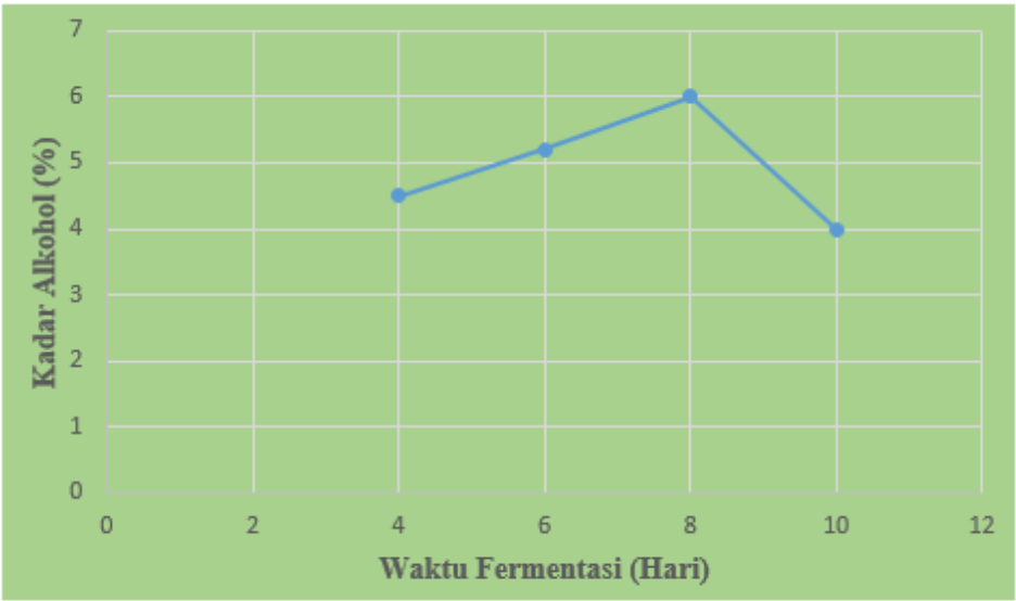
Grafik bioetanol hasil fermentasi kulit singkong. Sumber: Widyastuti, 2019
